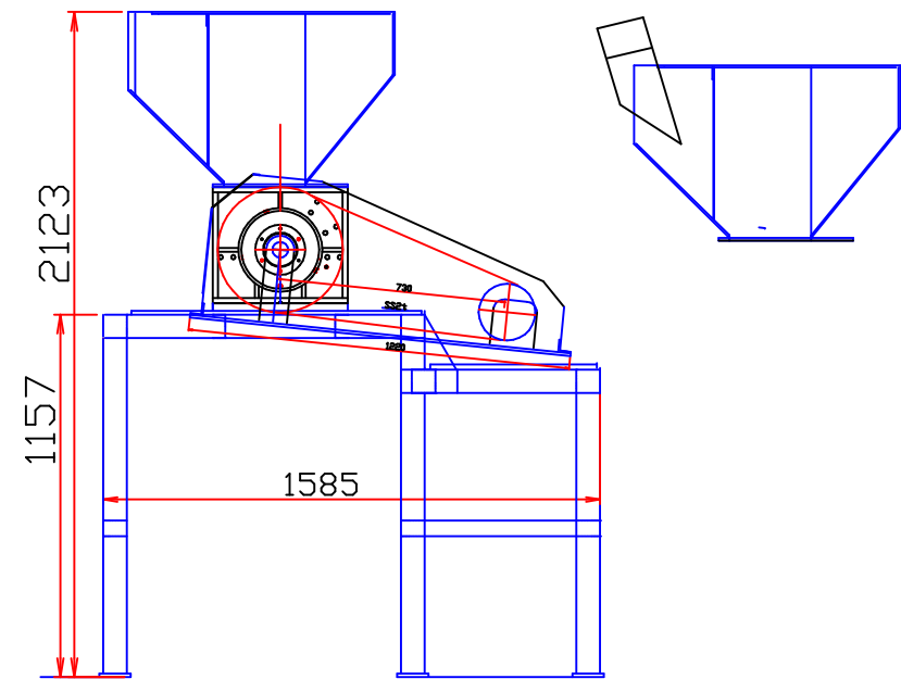
一次粉砕機
